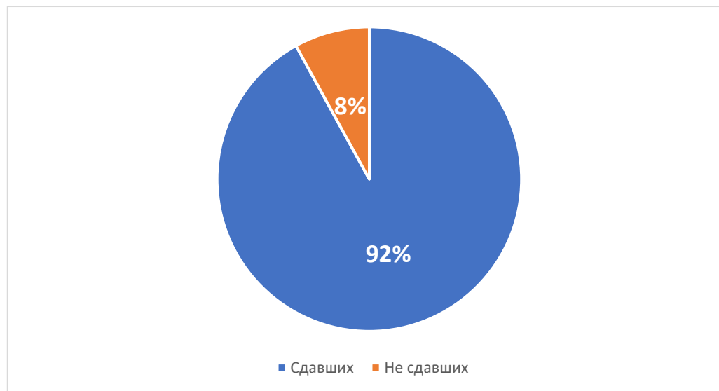
Средний % сдавших\не сдавших среди 2 курсов
