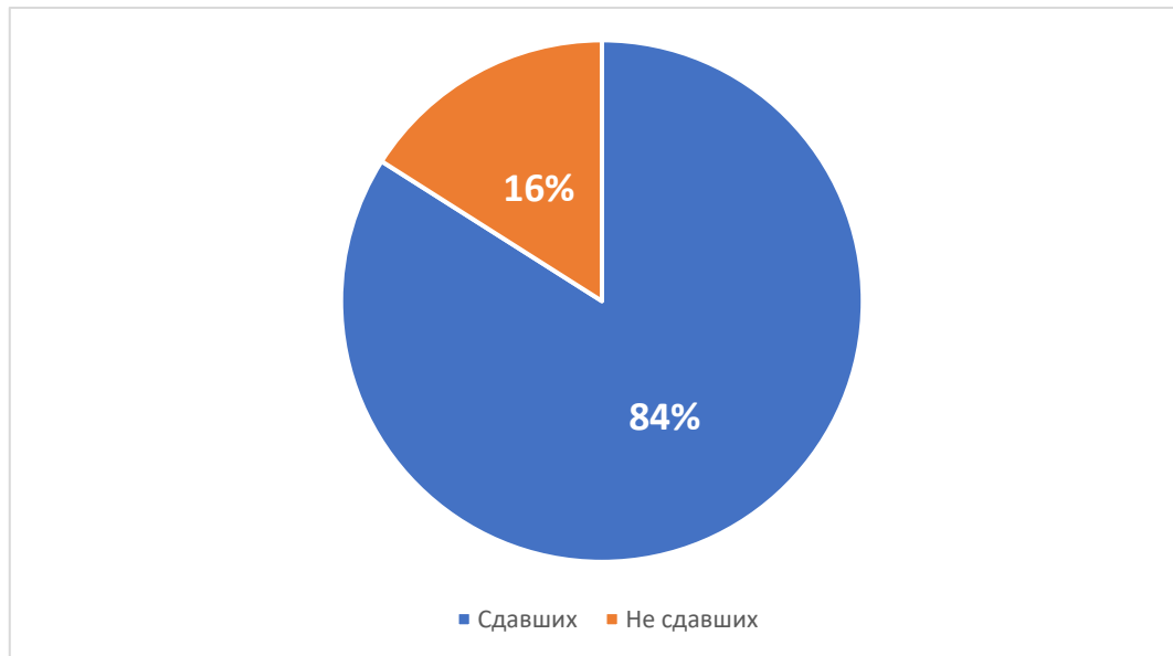
Средний % сдавших\не сдавших среди 4 курсов
