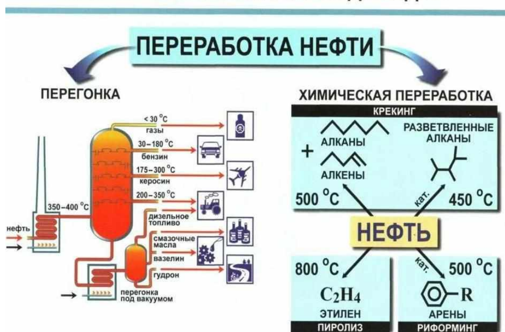
Рисунок 1 – Переработка нефти. Способы и технология переработки нефти
